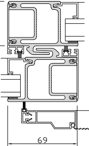
④ INTERLOCK STILE
